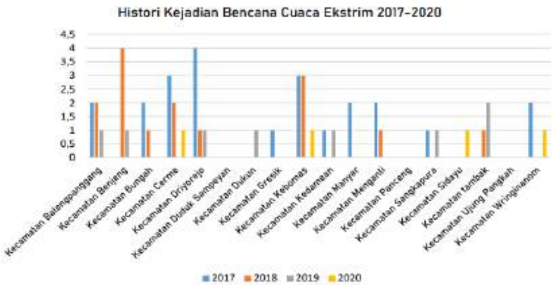
Gambar 2.5 Histori Kejadian Bencana Cuaca Ekstrem 2017 - 2020
