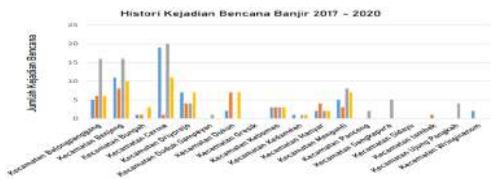
Sumber: KRB Kabupaten Gresik, 2021 Gambar 2.2 Histori Kejadian Bencana Banjir 2017 – 2020
