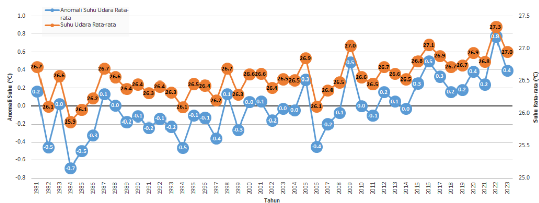
Gambar 3.2 Anomali dan Suhu Udara Rata Rata Indonesia
